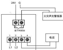
图 2 端子接线图
