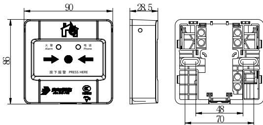
图 1 外形及尺寸图
